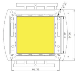
外光尺寸图
