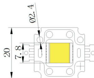
外光尺寸图
