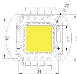
外光尺寸图
