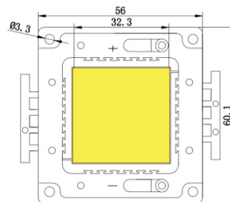
外光尺寸图
