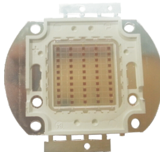
实物图
