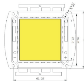
外光尺寸图
