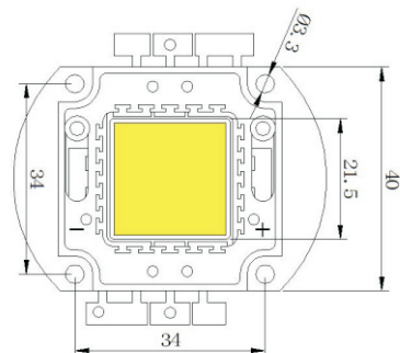
外光尺寸图
